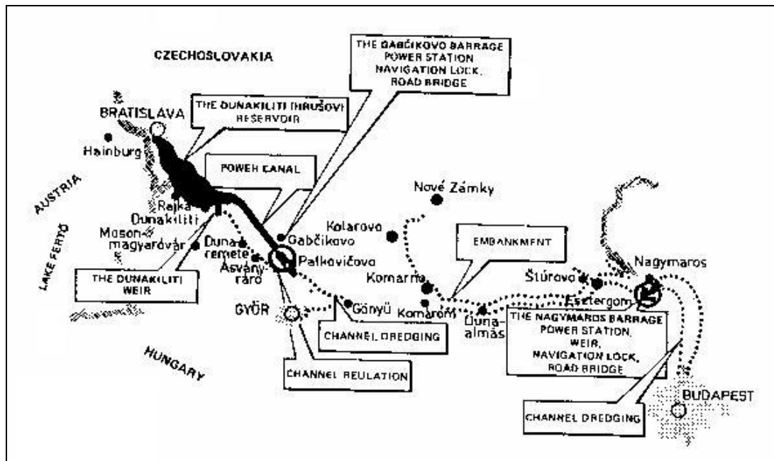
A Bős-Nagymarosi vízlépcsőrendszer áttekintő vázlata
